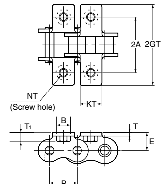
TYPE PK-1
